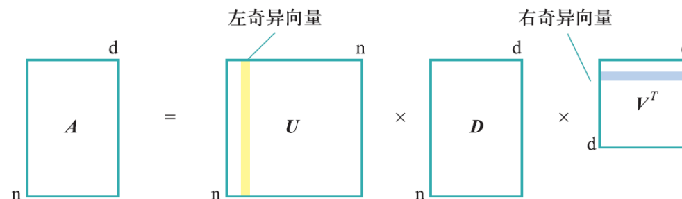
图 4.7 奇异值分解示意
